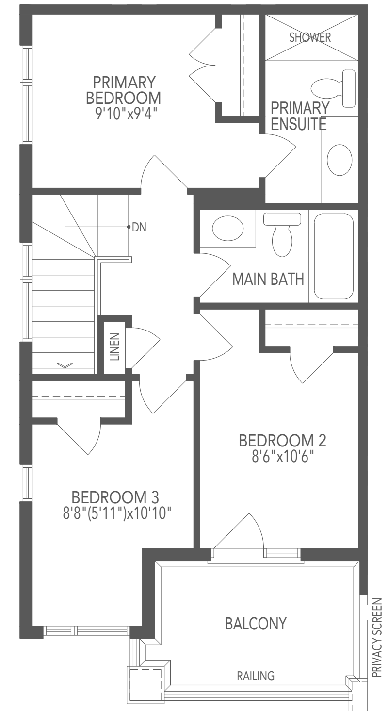
ELEV. A1
