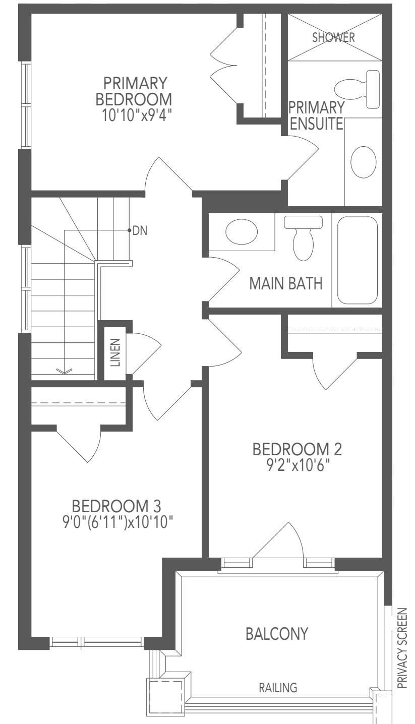
UPPER LEVEL ELEV. A1
